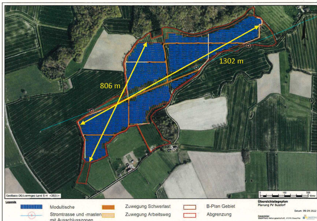
Abb. 1.2 Vorläufige Planung für die Errichtung der PVA Busdorf mit den Zuwegungsstrukturen (beige und ockerfarben), der Umzäunung (hellrote Linie) und den Trafostationen (kleine schwarze Rechtecke). Die geplante Fläche wird durch eine Freileitung (türkisfarbene Linie) in eine nördliche und eine südliche Hälfte geteilt (Quelle: Enertrag SE, Entwurf vom 09.09.2022). Die geplante PVA besitzt zwei Zerschneidungsachsen (gelbe Pfeile).
