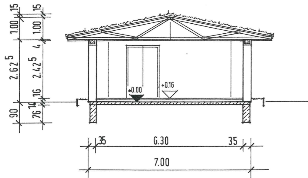
SCHNITT A-A'
